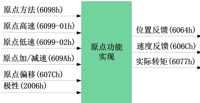
图 6.11 原点运动输入/出参数对象
