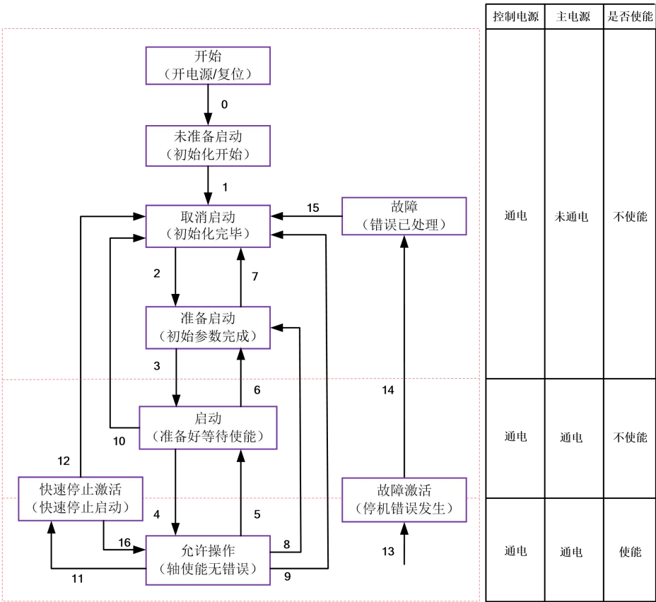
图 6.1 DM3B 的 402 状态机
