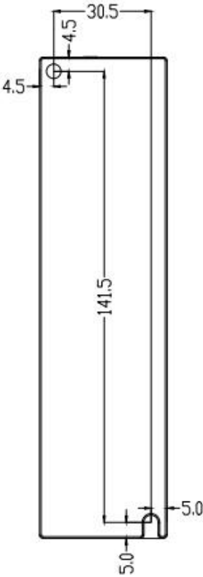
图 2-1 DM3B-EC882AC 安装尺寸图(单位：mm) ※ 设计安装尺寸时，注意考虑端子大小及布线！
