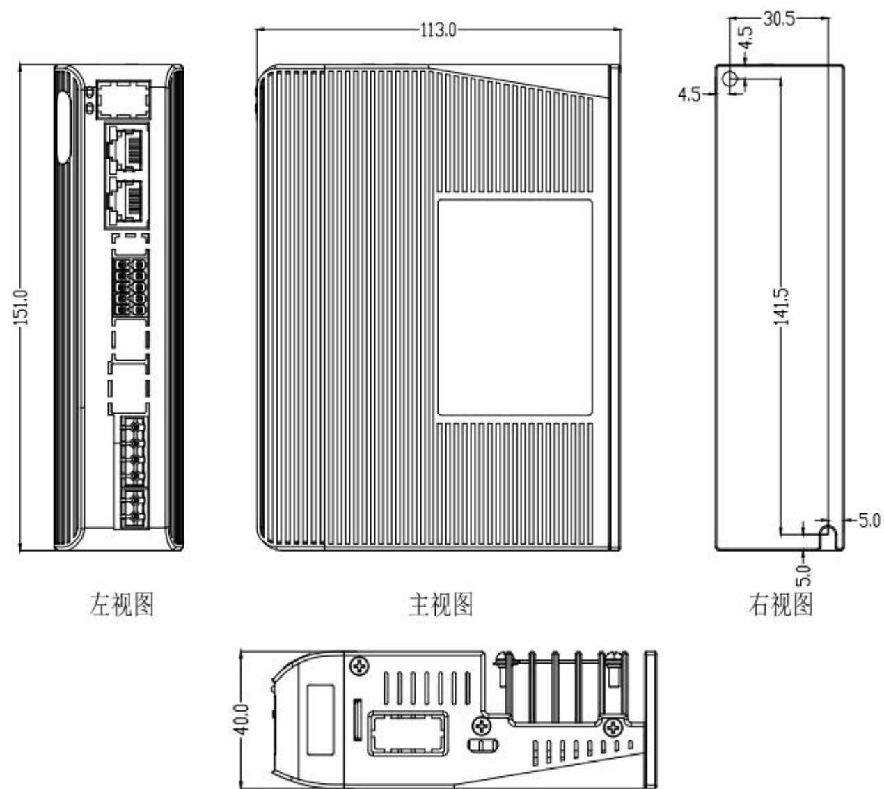
图 2-1 DM3B-EC882AC 安装尺寸图(单位: mm) ※ 设计安装尺寸时, 注意考虑端子大小及布线!
